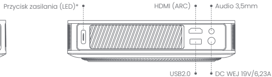
Widok z tyłu
